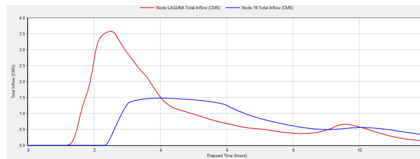
Figura 3: Caudal de entrada y salida espacio de laminación I, para la lluvia de 83mm
