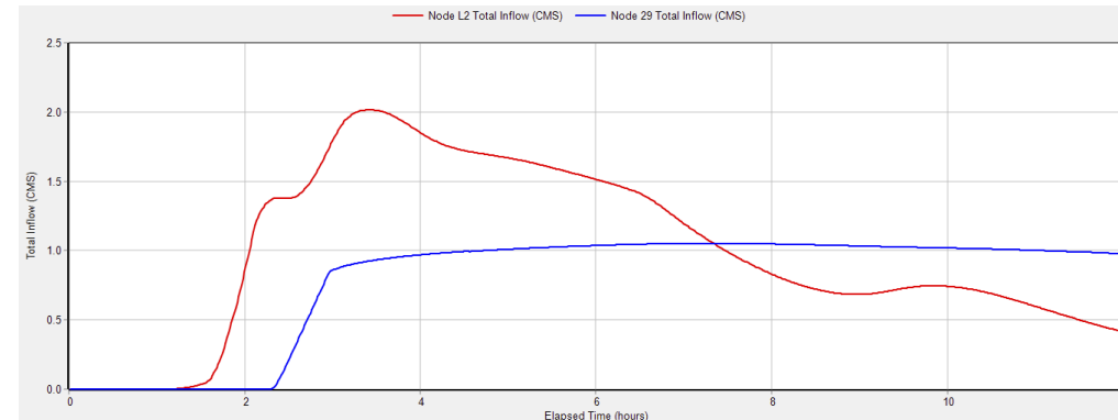
Figura 4: Caudal de entrada y salida espacio de laminación II, para la lluvia de 83mm
